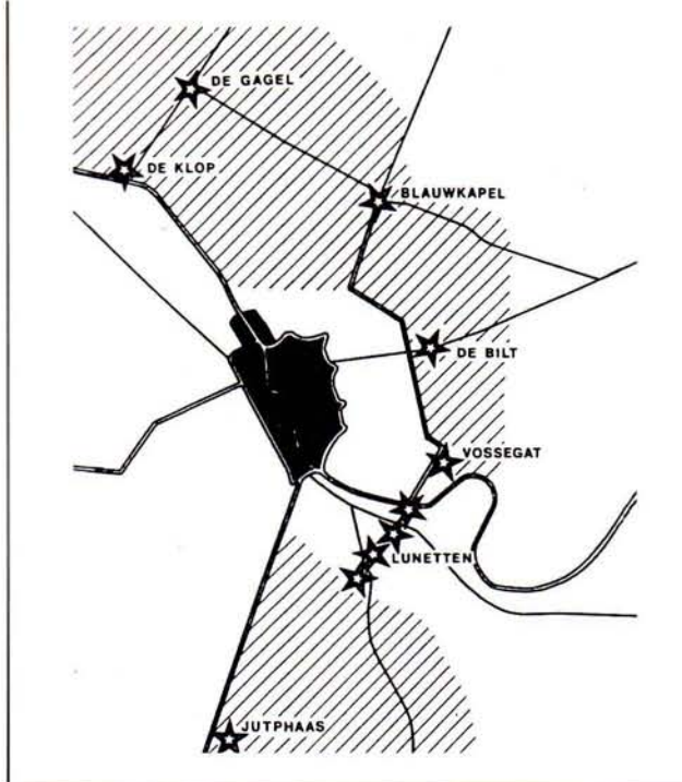
De door Willem Offerhaus gebouwde fortengordel rond Utrecht. Het gearceerde gedeelte kon worden geïnundeerd. (Naar G. Koppert, 'De forten rond Utrecht. Verdedigingswerken in de Nieuwe Hollandse Waterlinie', Utrecht 1983.)
